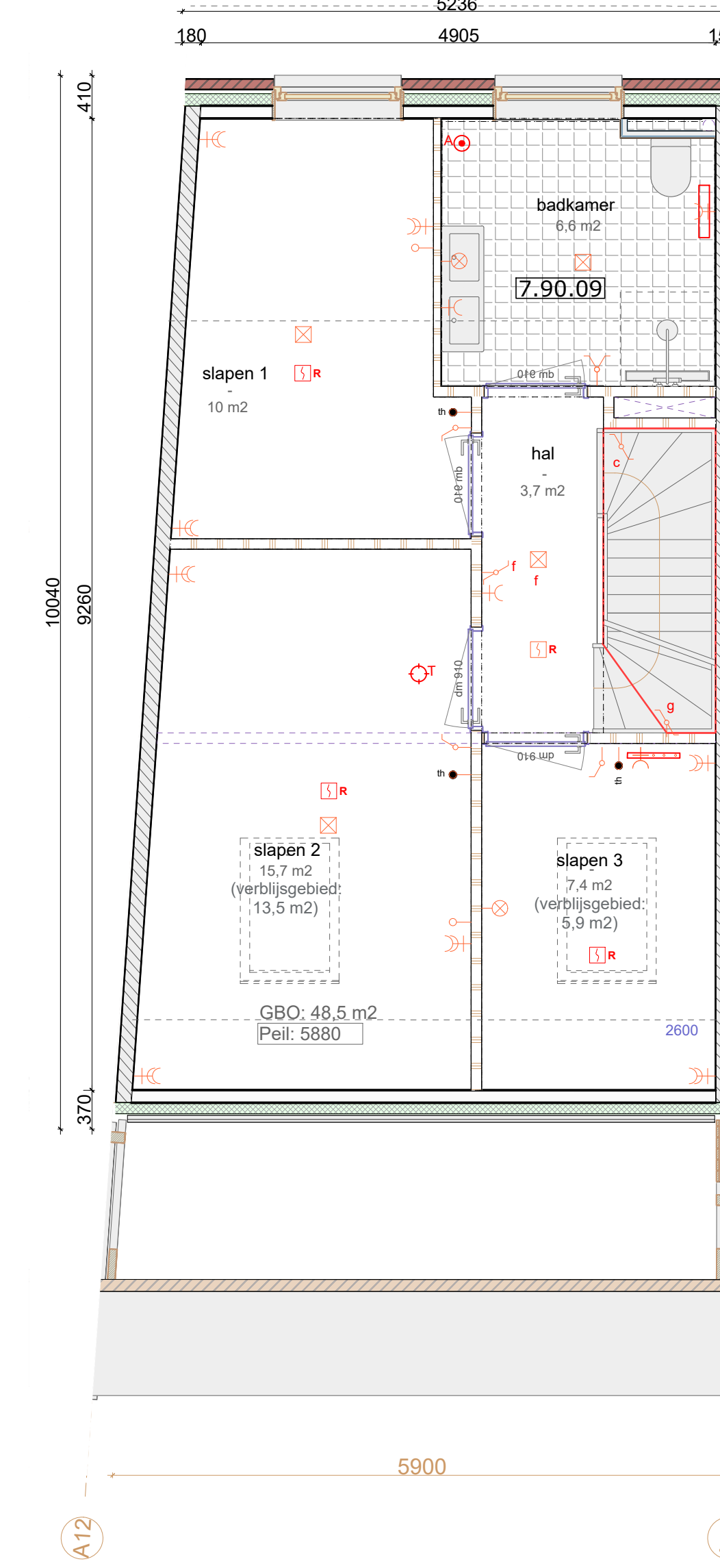
Tweede verdieping 1:50
