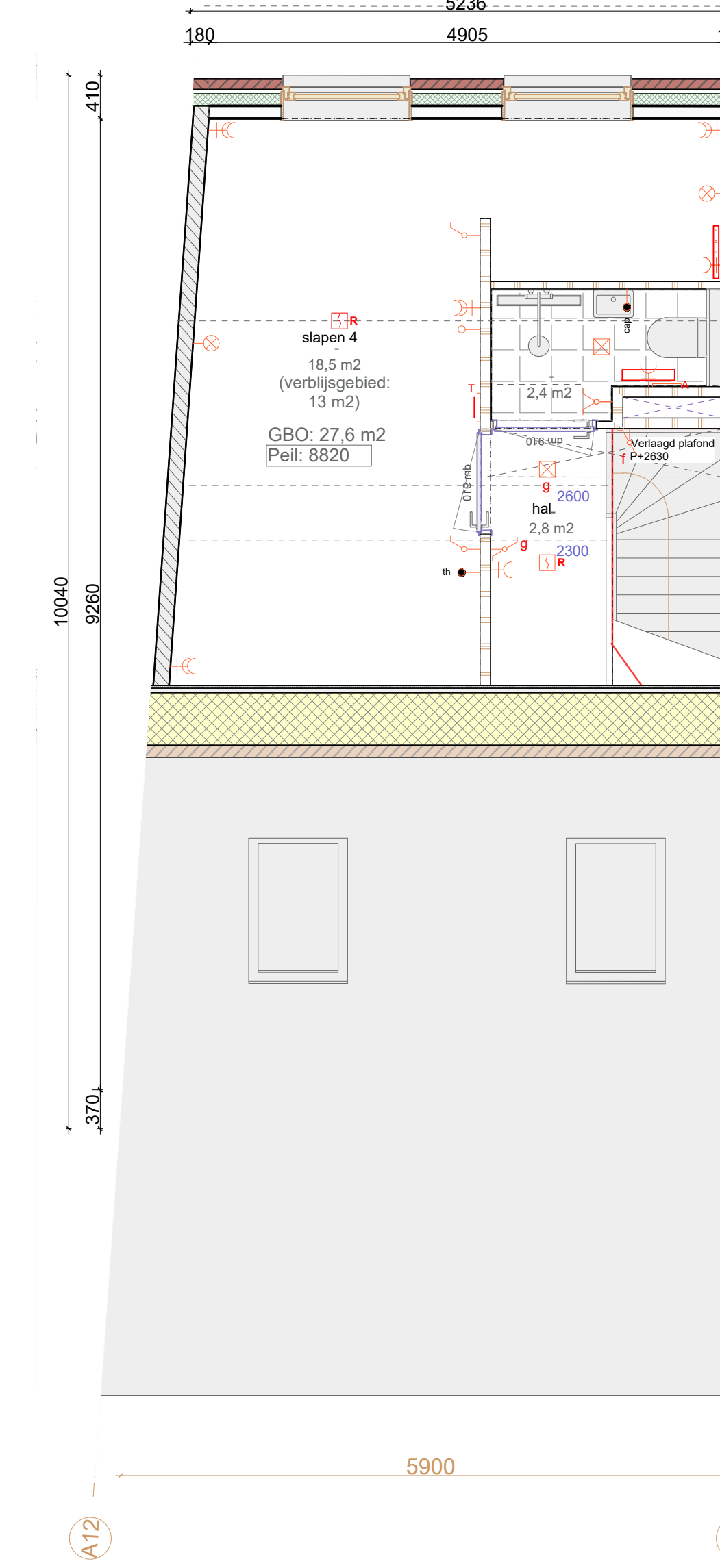
Derde verdieping 1:50
