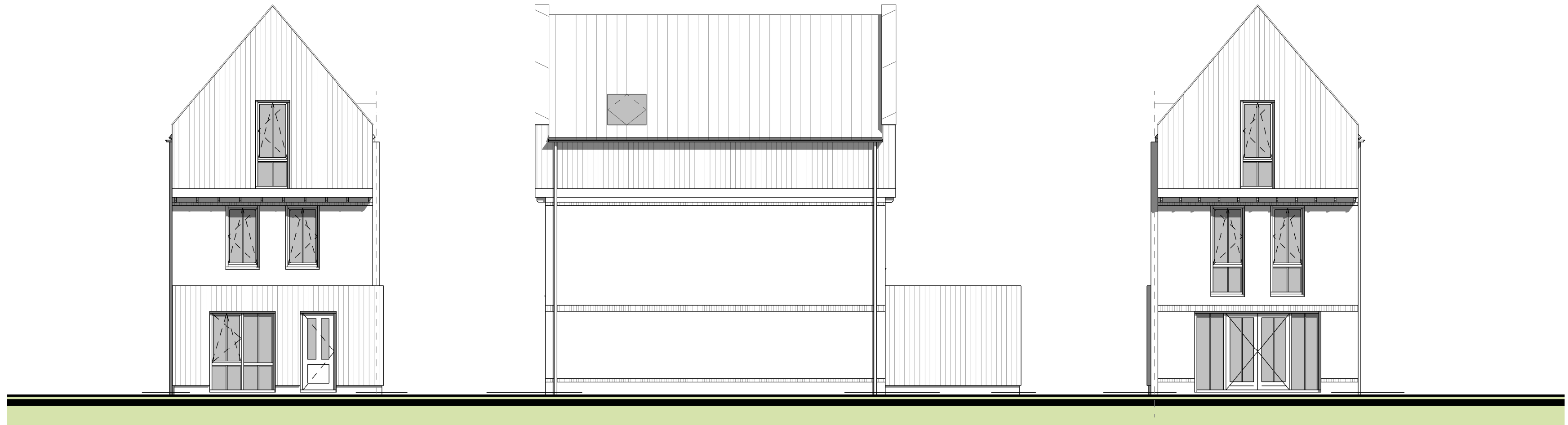
voorgevel 1.02 1 : 100
