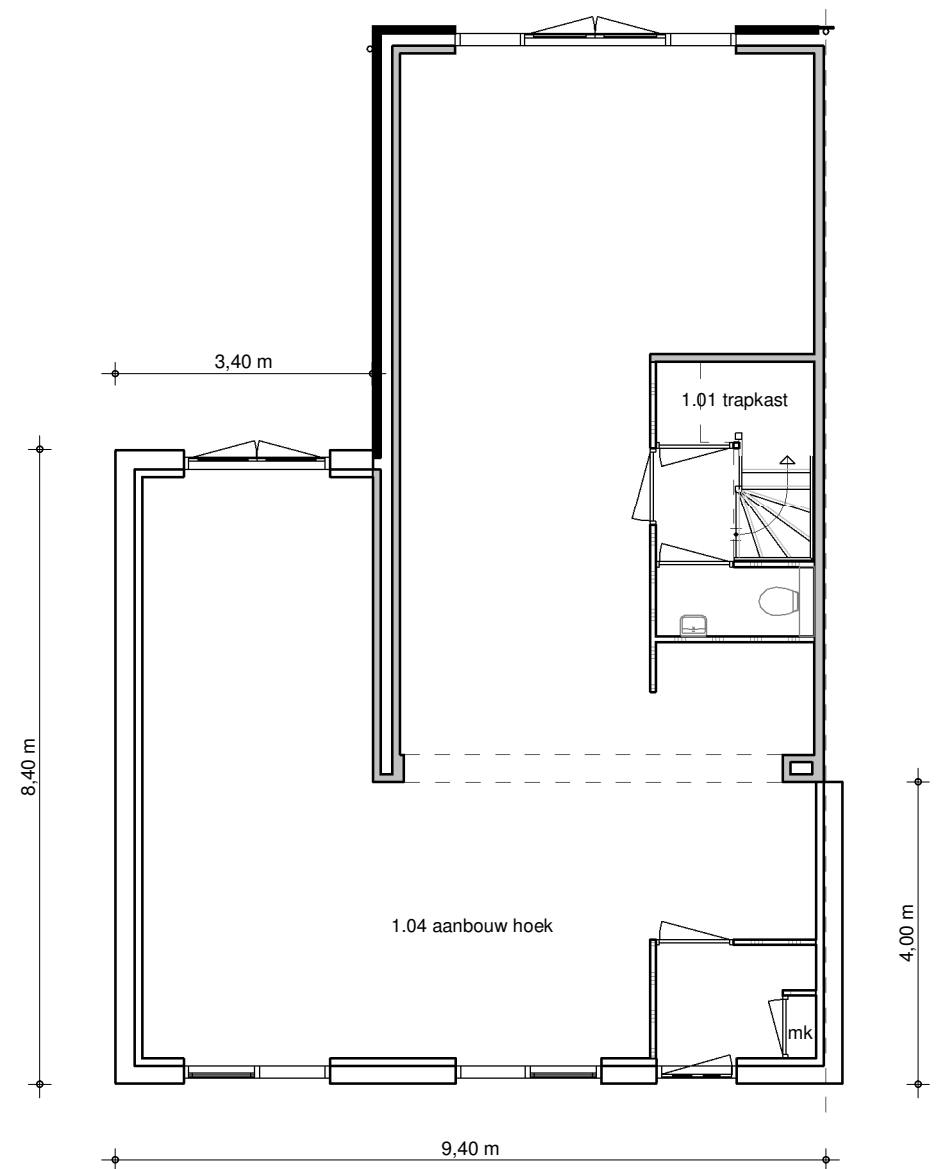
begane grond 1.04 1 : 100
