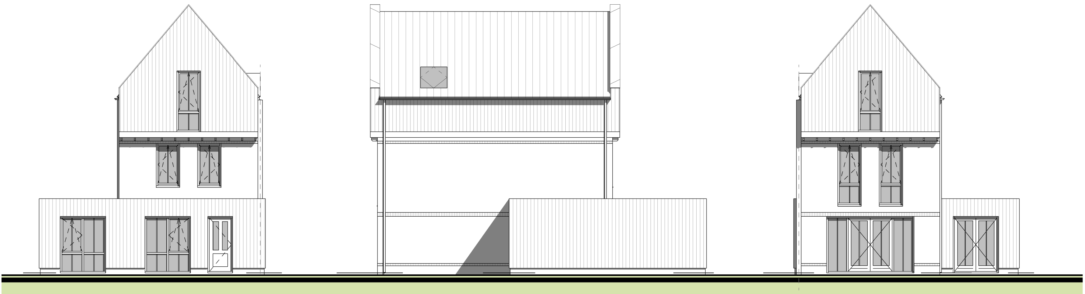
voorgevel 1.04 1 : 100
