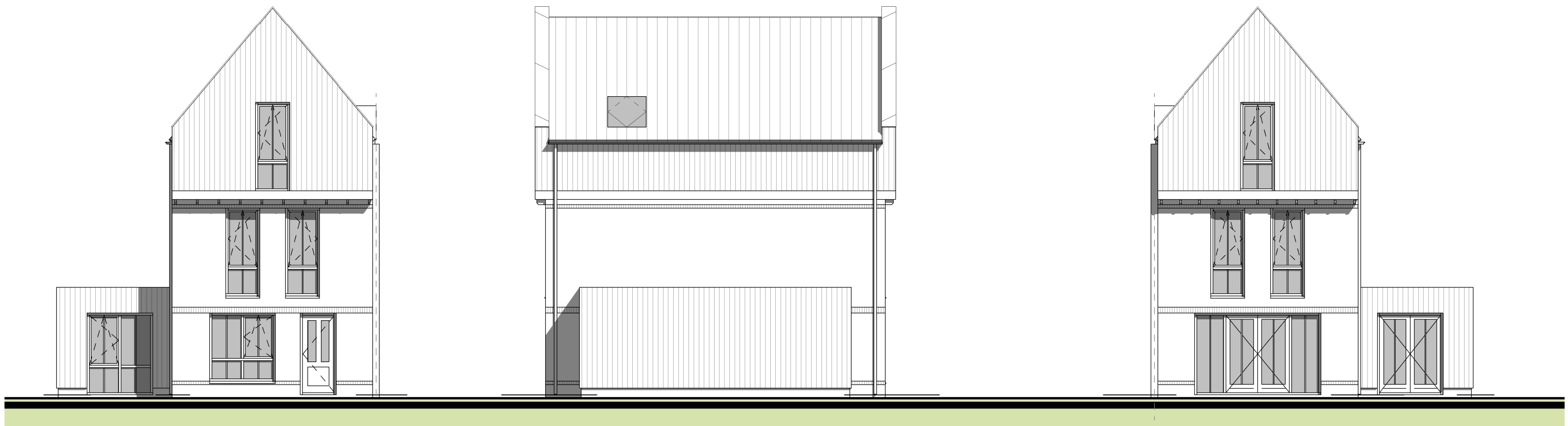
voorgevel 1.03 1 : 100
